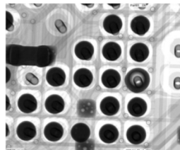
X-RAY 検査
